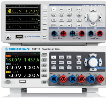
R&S®HMC8043 및 R&S®NGE100B 3채널 파워 서플라이
