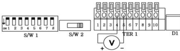
< 그림. 4-6 Remote Current Monitoring >
