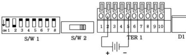
< 그림. 4-4 Remote Current Programming >
