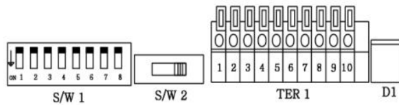
<그림. 4-2 Analog Control Terminal >
