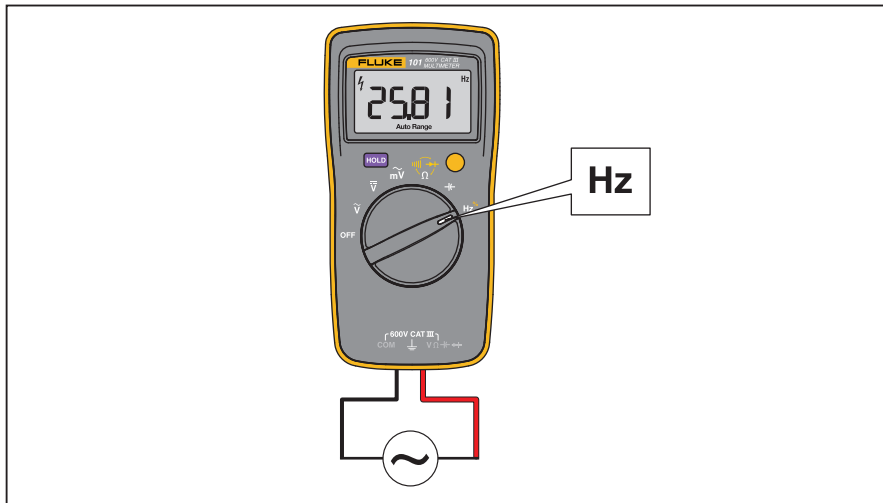
그림 4. 주파수 및 작동 사이클 측정
