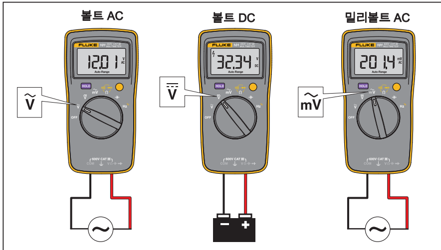
그림 2. AC 및 DC 전압 측정
