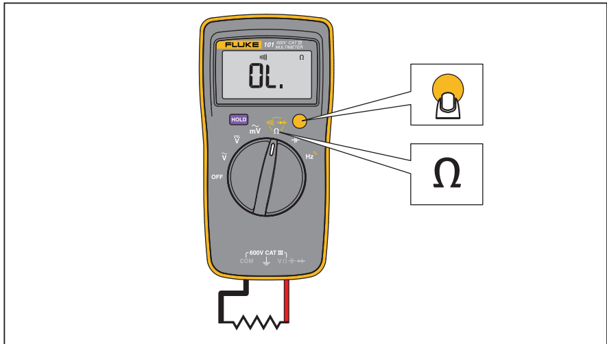
그림 3. 저항/연속성 측정
