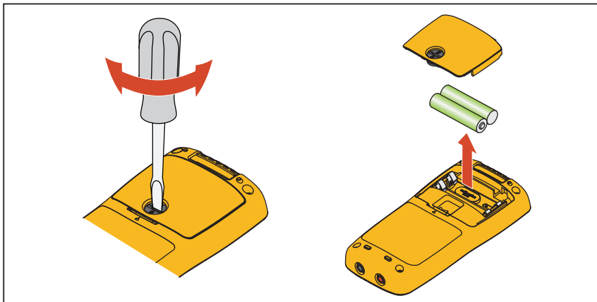
그림 5. 배터리 교체
